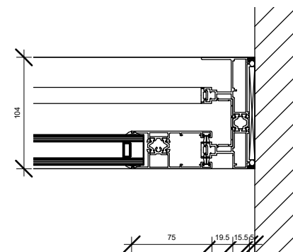
5 Detail 3 1 : 5
