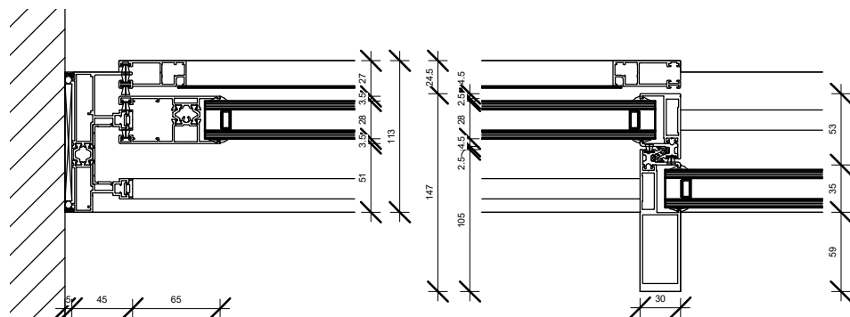
3 Detail 1 1 : 5
