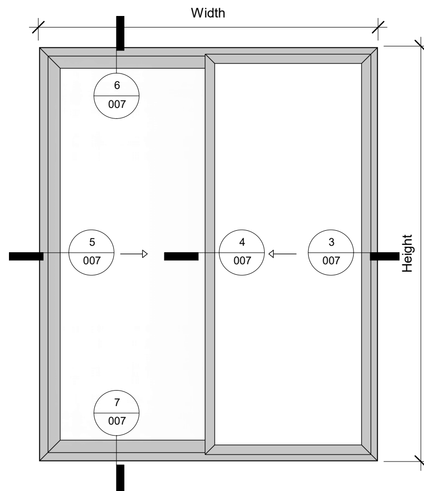
2 Elevation Back 1 : 20
