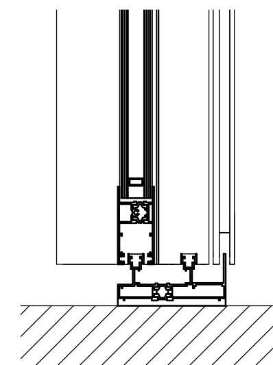
7 Detail 5 1 : 5
